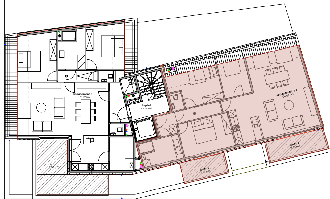
PLAN VERDIEPING 3 schaal 1-200
